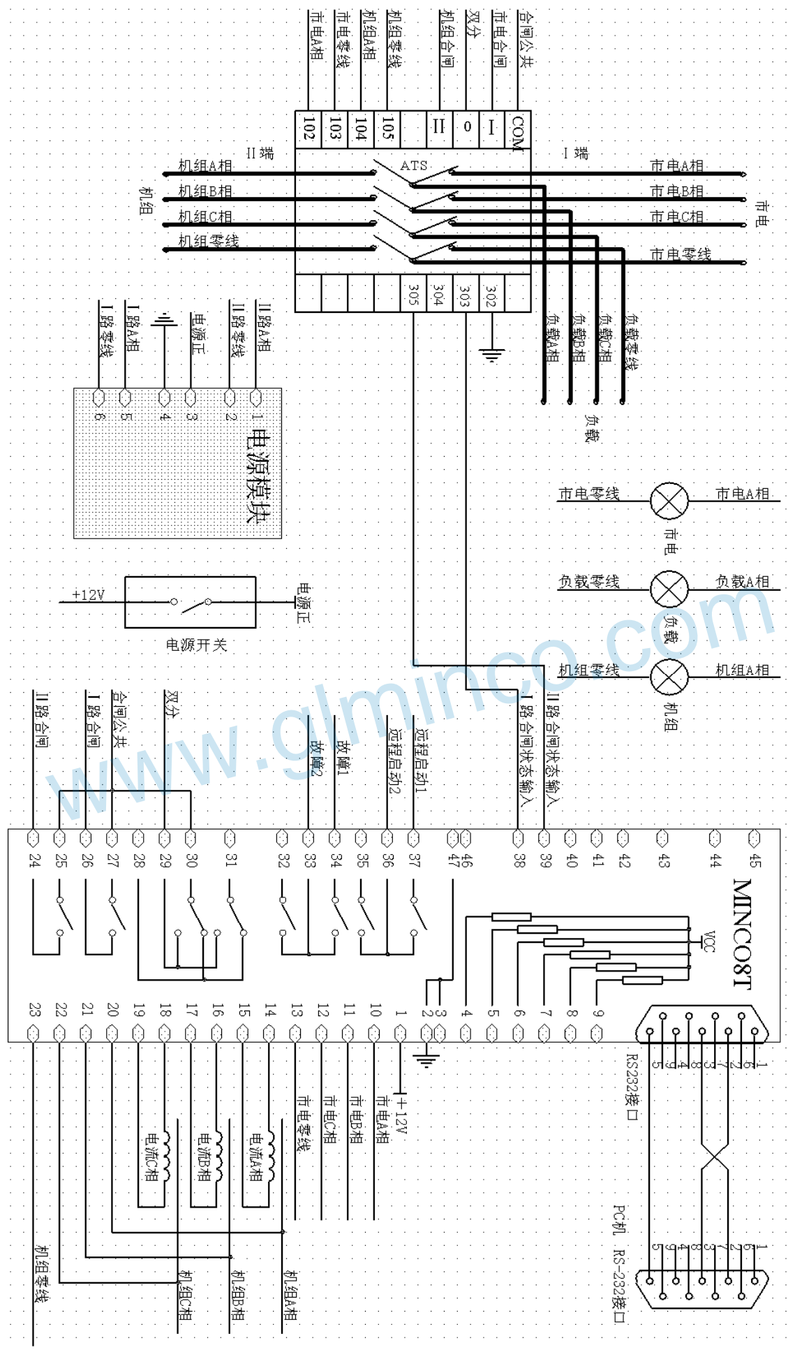
MINCOST双路电源自动切换控制器接线图
